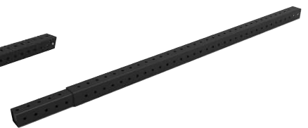
PA 55075400 Columna alargador. 180 cm. Medida total 207 cm con alargador. Peso: 13.5 kg.
