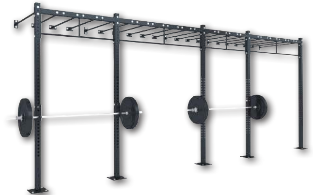
PA 55087800 Estructura Funcional C9. Medidas: 577 x 112 x 275 cm. PA 55088800 Estructura Funcional D9. Medidas: 577 x 172 x 275 cm.
